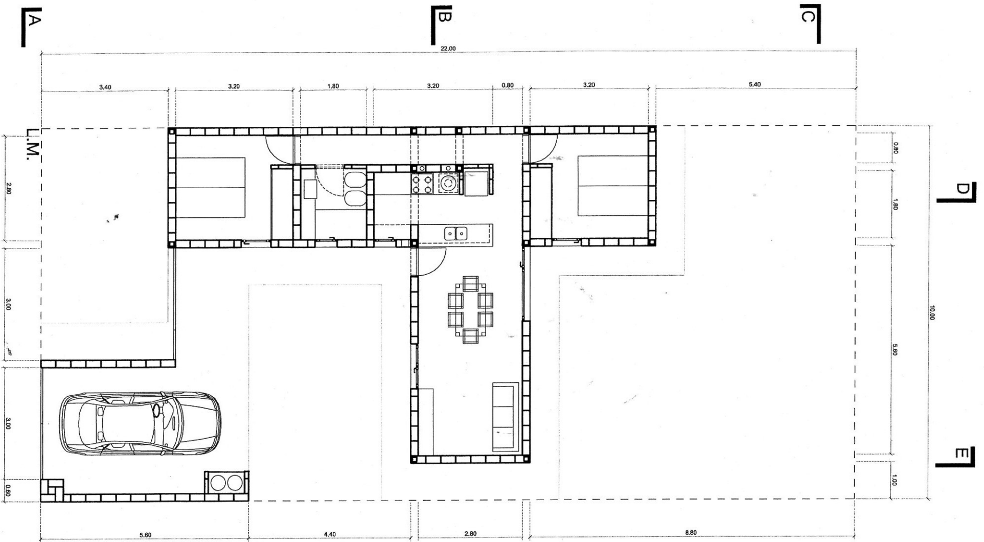
PLANTA 2 HABITACIONES 58,60m 2
